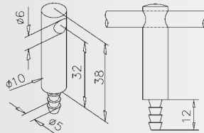
„Mini rail“ Centre bracket for mounting on wood Mittelstütze für Holzmontage Support traversant, fixation sur bois Middensteun voor montage op hout
