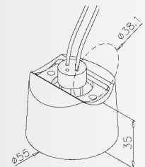
Tube lamp connector Halogenstrahler (Rohraufsatz) Spot halogène Halogeenspot (opbouw)
