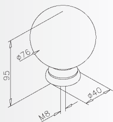
Universal angle ball Endkugel Bouton d'ornement Eindbol
