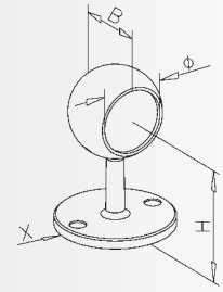
Ball end post Rohrendhalter Support borgne Opschuij eindsteun
