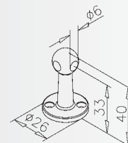
Mini-fiddle rail elbow bracket 90° Eckstütze 90° Raccord d'angle 90° Hoeksteun 90°
