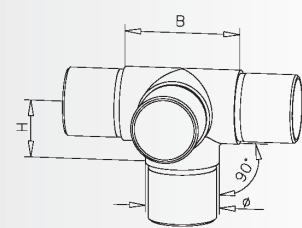
Flush tee + 1 outlet 90° Rohrverbinder T + 1 Abzw. 90° Raccord en T + 1 départ 90° T-fitting + 1 uitg. 90°
