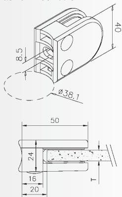
Glass clamp for tube Glasklemme für Rohr Pince à verre pour tube Glasklem voor buis
