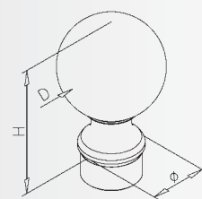
Ball top Endkugel Bouton d'ornement Eindbol
