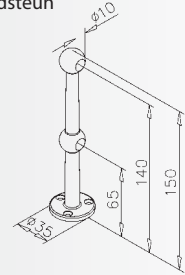
Double fiddle rail end bracket Doppelte Endstütze Double support borgne Dubbele eindsteun
