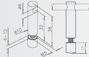
„Mini rail“ Centre bracket for mounting on glass Mittelstütze für Glasmontage Support traversant, fixation sur verre Middensteun voor montage op glas
