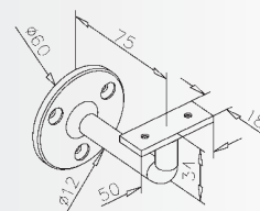
Flat handrail bracket Handlaufstütze flach Support main-courante plat Vlakke leuninghouder
