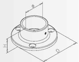
Wall and floor flange Wand- und Bodenflansch Embase Muur en vloer flens
