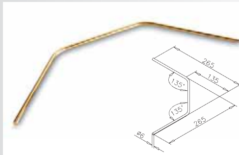
„Mini rail“ Rod 2 x 135° Stab 2 x 135° Barre 2 x 135° Staf 2 x 135°
