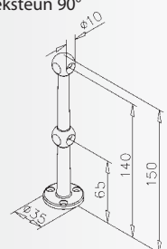
Double fiddle rail elbow bracket 90° Doppelte Eckstütze 90° Double raccord d'angle 90° Dubbele hoeksteun 90°
