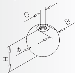
End ball Zierkugel Bouton d'ornement Sierkugel
