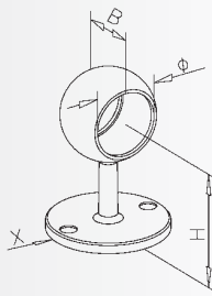
Ball centre post Rohrhalter Support traversant Opschuijsteun
