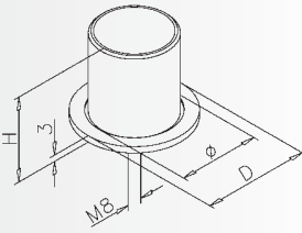
Tube connector Rohrbefestigungshülse Embase manchon Buis bevestigingsflens
