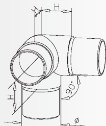
Flush elbow 90° + 1 outlet 90° Rohrverbinder 90° + 1 Abzw. 90° Raccord coude 90° + 1 départ 90° Kniefitting 90° + 1 uitg. 90°
