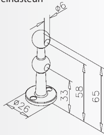
Double mini-fiddle rail end bracket Doppelte Endstütze Double support borgne Dubbele eindsteun
