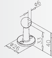
Mini-fiddle rail end bracket Endstütze Support borgne Eindsteun
