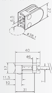
Glass clamp for tube Glasklemme für Rohr Pince à verre pour tube Glasklem voor buis
