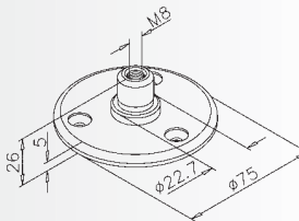
Base flange Innenflansch Embase manchon Combinatie flens
