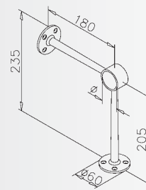
Floor bracket Fußlaufstütze Support repose-pied Voetsteun
