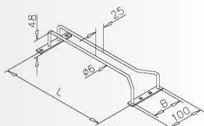
Glass rack Gläserhalter Support à verres Glazenhouder
