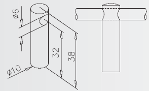
„Mini rail“ Centre bracket for glue fixation Mittelstütze für Klebemontage Support traversant, fixation avec colle Middensteun voor lijm montage
