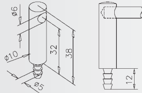
„Mini rail“ End bracket for mounting on wood Endstütze für Holzmontage Support borgne, fixation sur bois Eindsteun voor montage op hout
