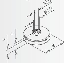
Finial with M8 Zier-Abschlusscheibe Embout de finition fileté Sier afsluitkap
