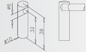
„Mini rail“ End bracket for glue fixation Endstütze für Klebemontage Support borgne, fixation avec colle Eindsteun voor lijm montage
