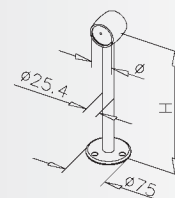
Adjustable floor bracket Fußlaufstütze variabel Support repose-pied variable Variabele voetsteun
