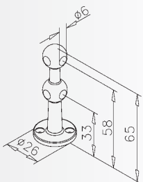
Double mini-fiddle rail elbow bracket 90° Doppelte Eckstütze 90° Double raccord d'angle 90° Dubbele hoeksteun 90°
