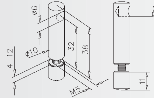
„Mini rail“ End bracket for mounting on glass Endstütze für Glasmontage Support borgne, fixation sur verre Eindsteun voor montage op glas
