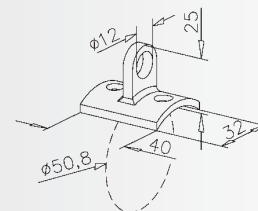
Tube plate Rohrauge Oeilleton pour tube Buisoog
