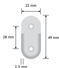
ALU KASTBAARHOUDER OVAAL OPEN.
